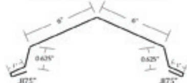
# 302 Reg Ridge S. Seam
