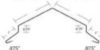
# 307 Wide Ridge S. Seam
