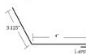
# 404 Reg S. Seam Head Wall
